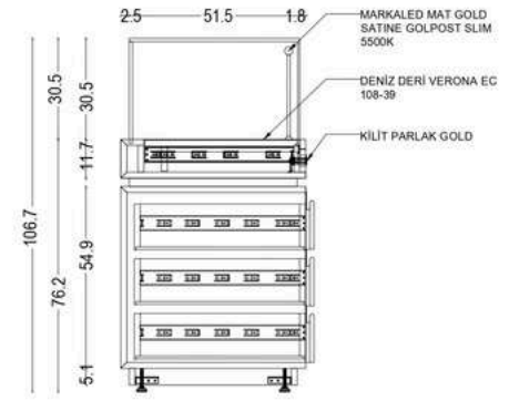
2 SECTION A-A
