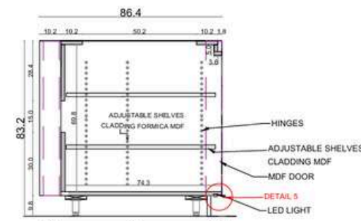
A-A SECTION
